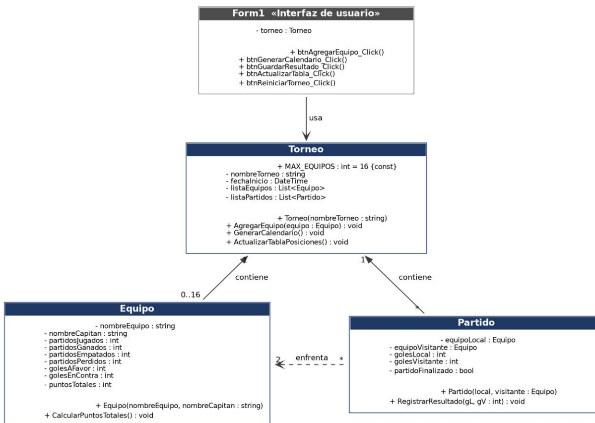
Figura 1. Diagrama de clases de Gestor de Torneos Locales.
